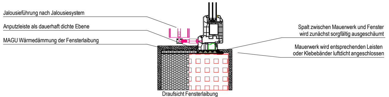
Draufsicht Fensterlaibung
